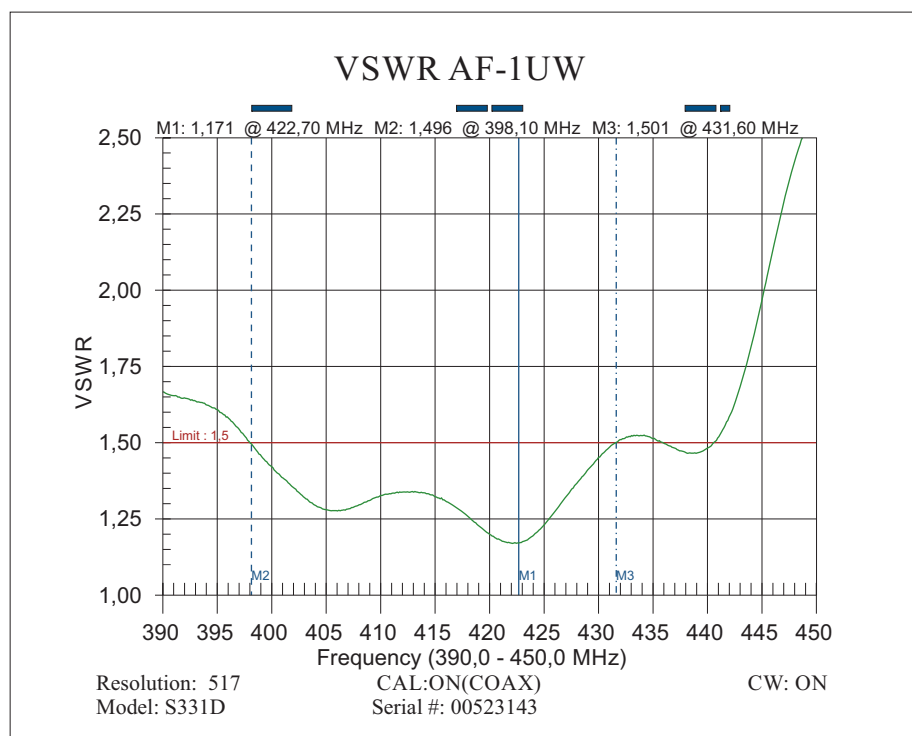
Типовое КСВ для F(C)=422,7 МГц
