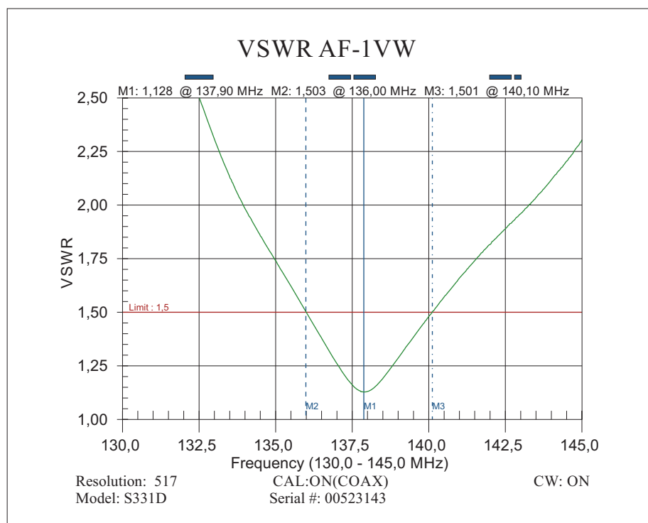
Типовое КСВ для F(C)=137,9 МГц
