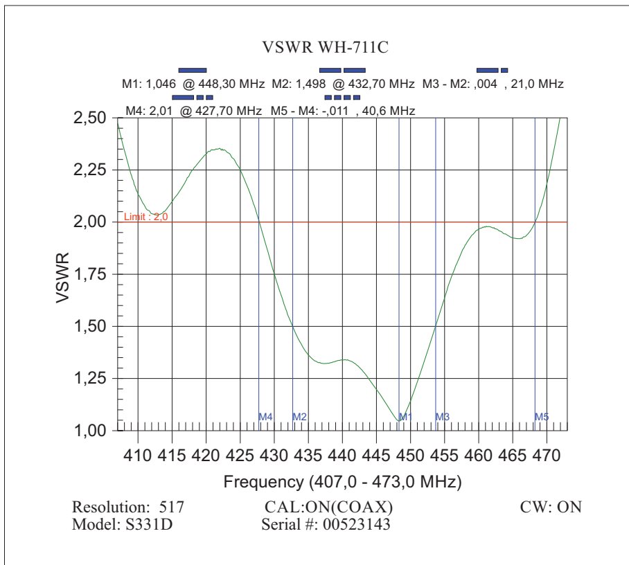
Типовое КСВ для F(C)=448,3 МГц на креплении MC-1 UHF
