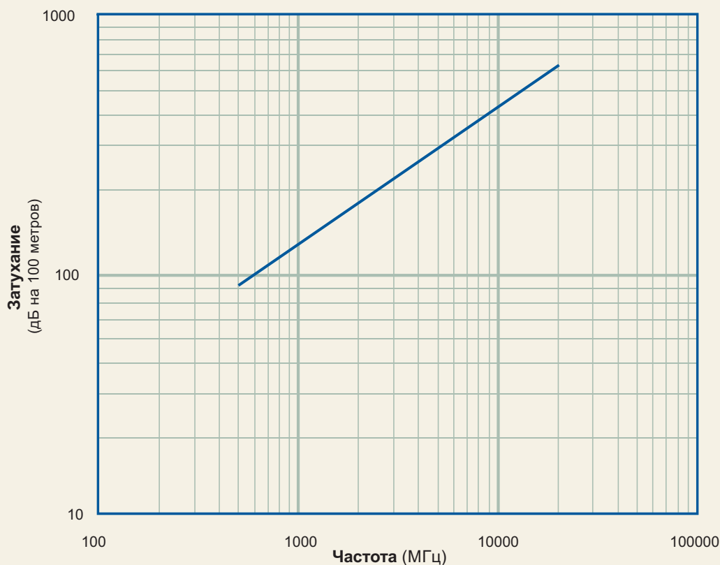
Типовое затухание SF-047 ST
