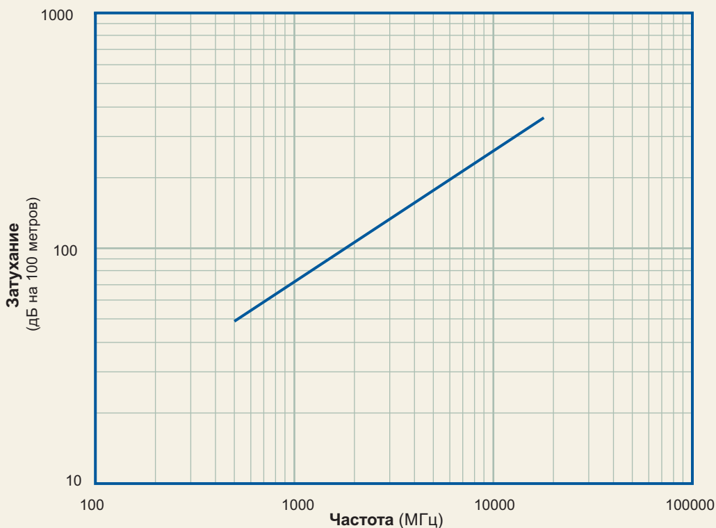
Типовое затухание SF-085/086 ST FEP
