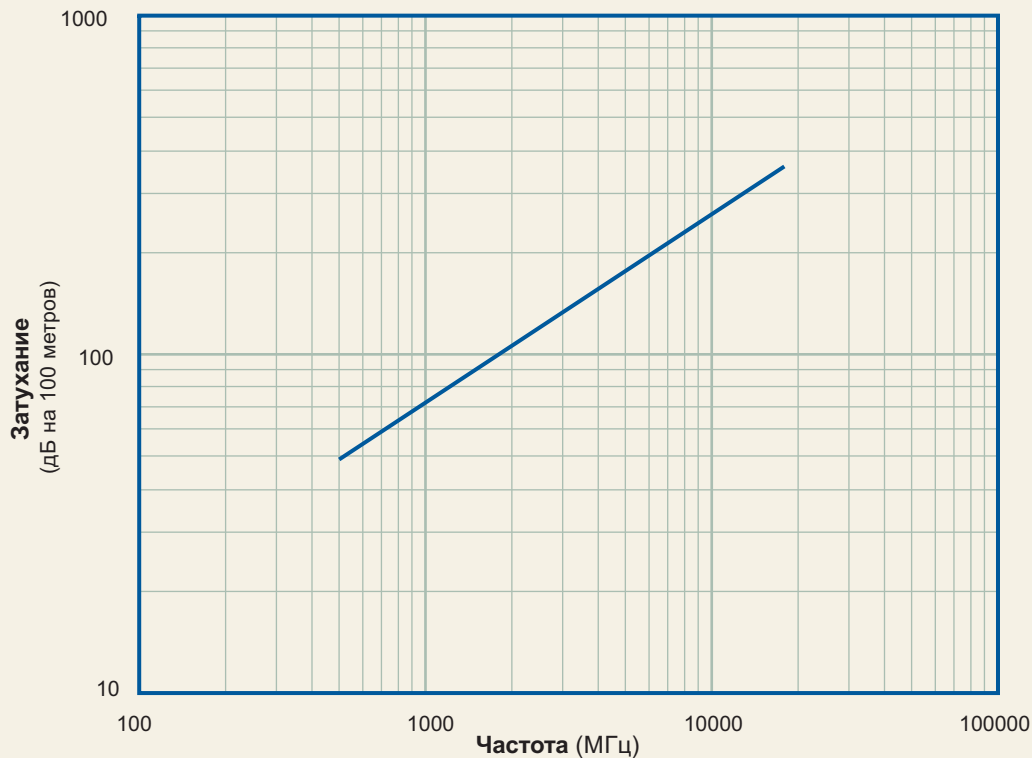
Типовое затухание SF-086 ST
